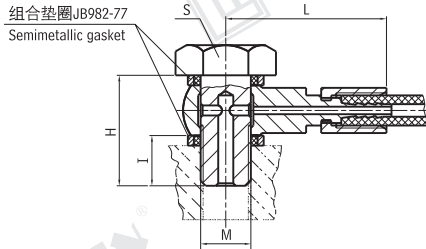
1、铰接式 Adjustable fitting: HF J ※ 单位 Unit:mm
