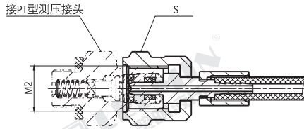
3、快换式 Quick fitting: HFH ※ 单位 Unit:mm
