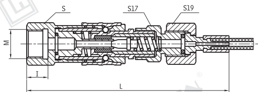
7、速换式 Snap-check fitting: HFS ※ 单位 Unit:mm
