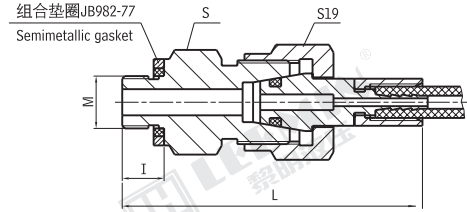
2、锥面密封式 Cone seal fitting: HF 0 ※ 单位 Unit:mm
