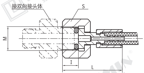
6、外固定螺纹式 Outor fixed thread: HFG ※ 单位 Unit:mm
