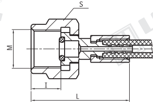
4、直接接压力表 Direct connect to pressure gauge: HFP ※ 单位 Unit:mm
