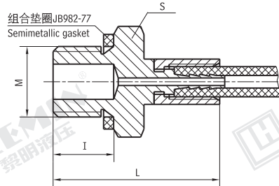
8、外螺纹式 Outer thread HFE ※ 单位 Unit:mm
