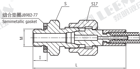
5、卡套式 Tube jam fitting: HFK ※ 单位 Unit:mm
